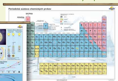
Periodická sústava chemických prvkov
